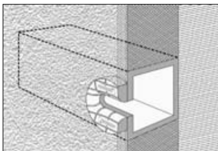
Schematický náčrt budky, instalované ve vrstvě zateplení v atikovém prostoru objektu v místě stávajících VO
